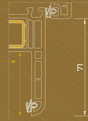
IGLO ENERGY CLASSIC TELAIO RISTRUTTURAZIONE 47 mm
