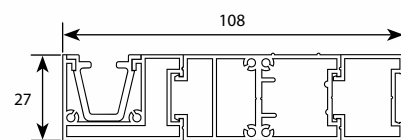
guida singola con sfalsamento
