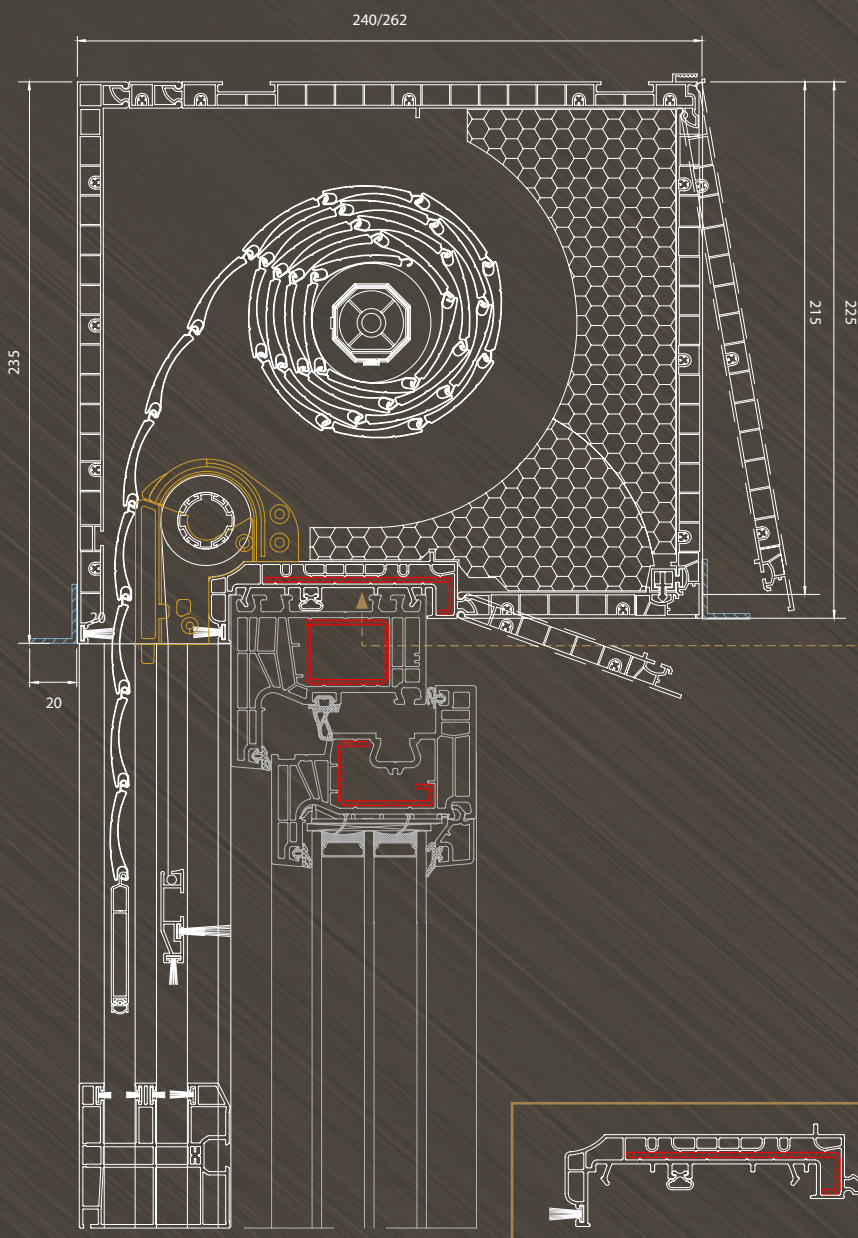
adattatore con rinforzo
