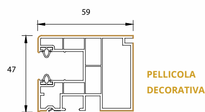
guida monolaterale
